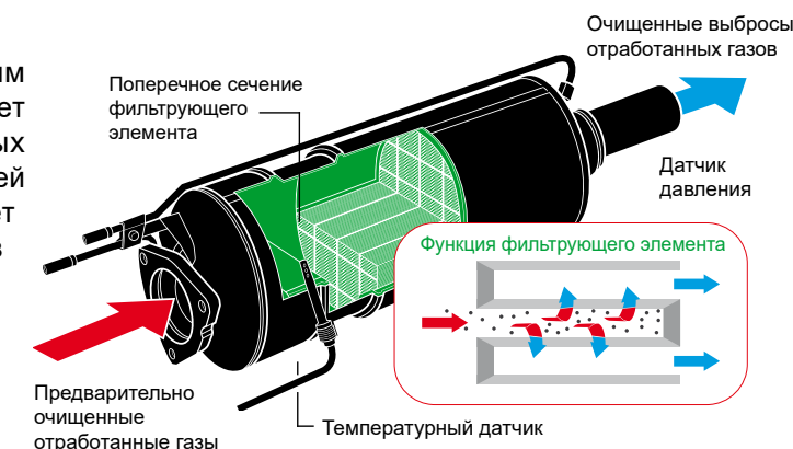
Обычное функционирование современного дизельного противосажевого фильтра
